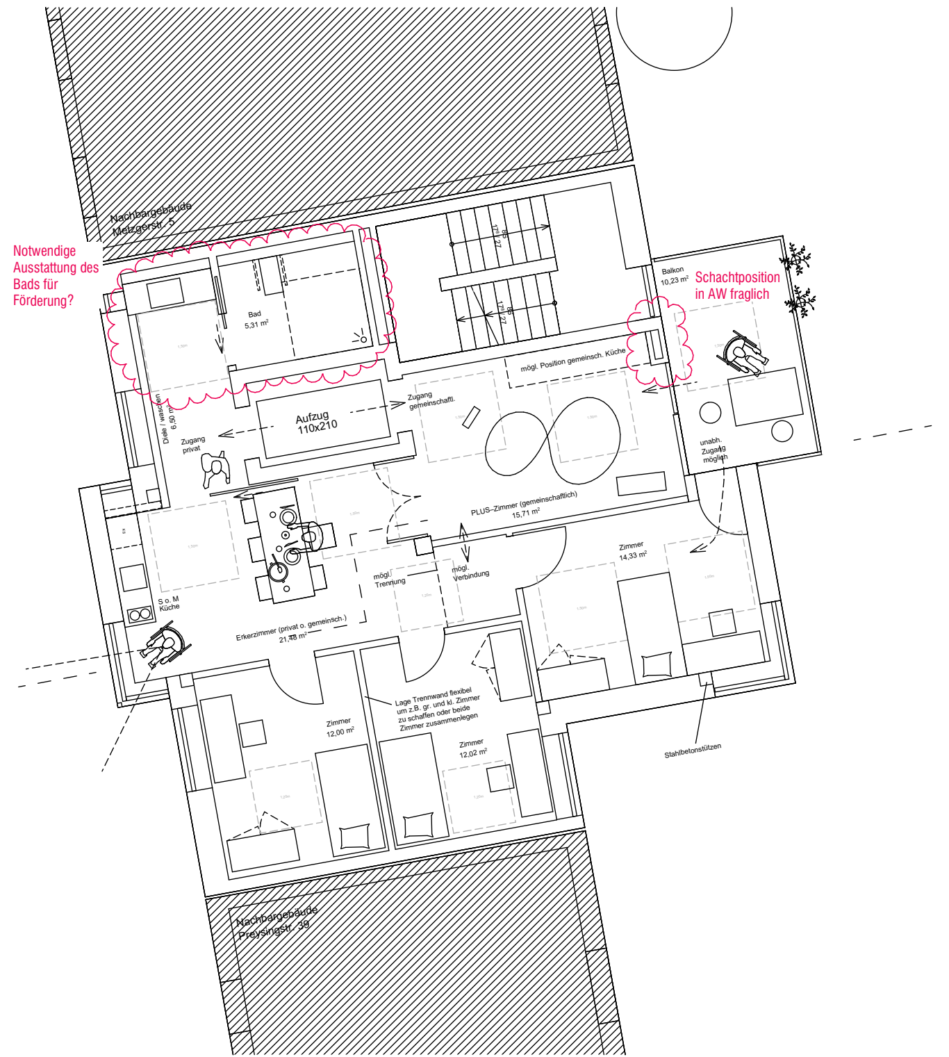
2.Obergeschoss
