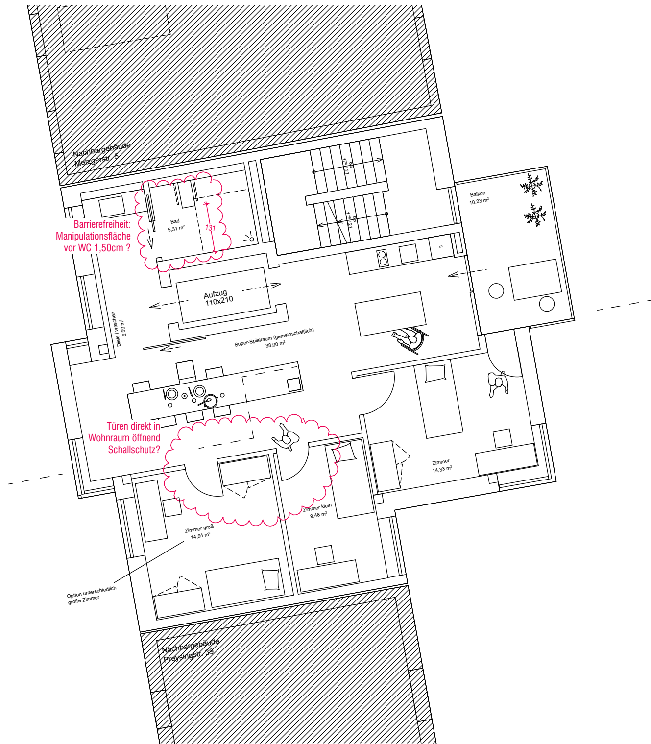
3.Obergeschoss
