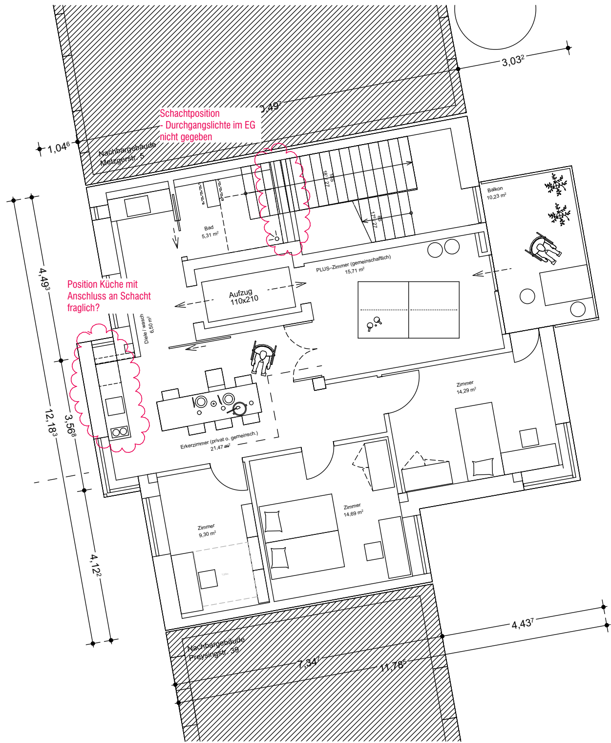
1.Obergeschoss
