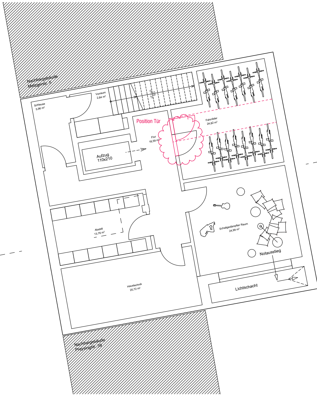
Untergeschoss
