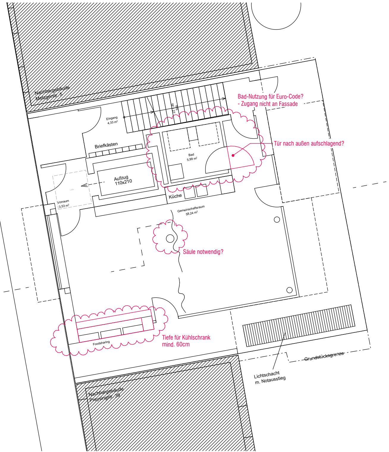
Erdgeschoss
